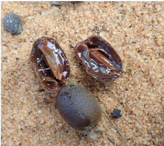
Fruits et graines de Diospyros latispatulata H. Perrier
