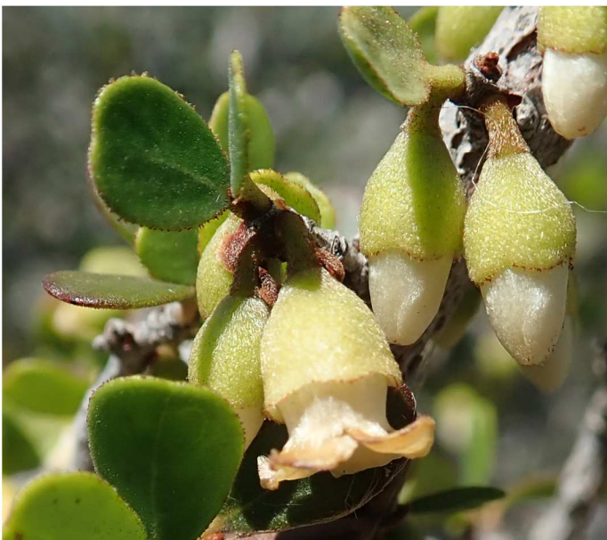
Diospyros manampetsae H. Perrier
