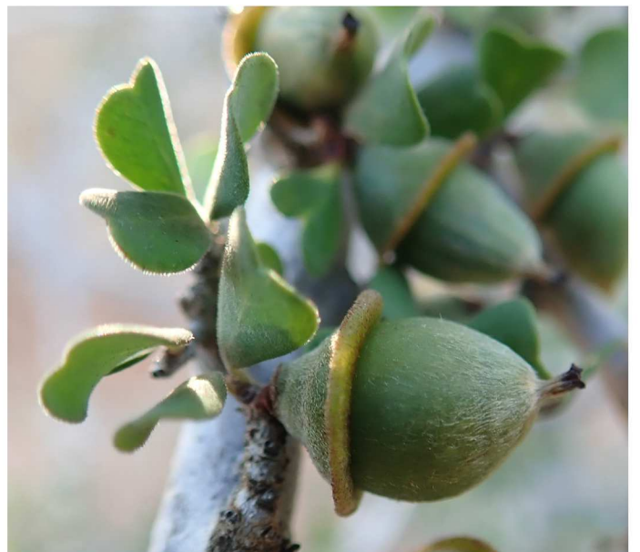
Diospyros manampetsae H. Perrier
