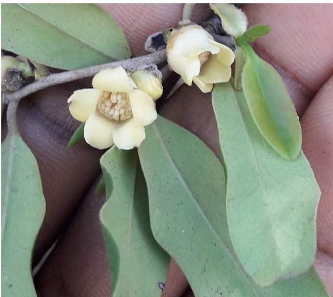
Diospyros cupulifera H. Perrier - Bibilaby
